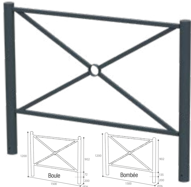
Version tête bombée
