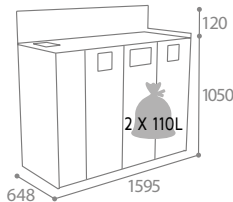
■ Réf. 53871 - Compact HPL Anthracite
